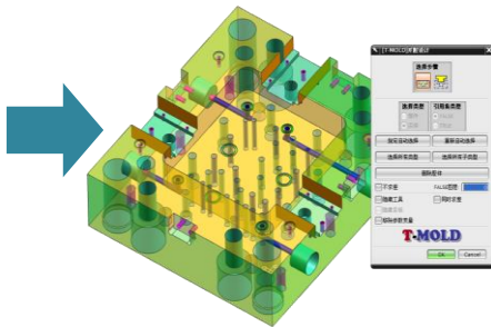
一键开腔
